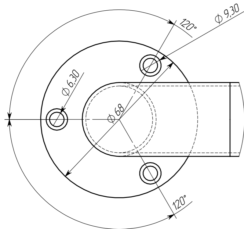
ВИД А МАСШТАБ 1 : 1
