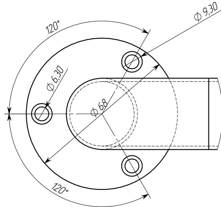
ВИД А МАСШТАБ 1 : 1
